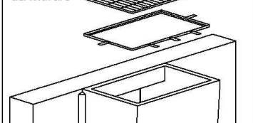
Grata rimovibile con telaio da murare
