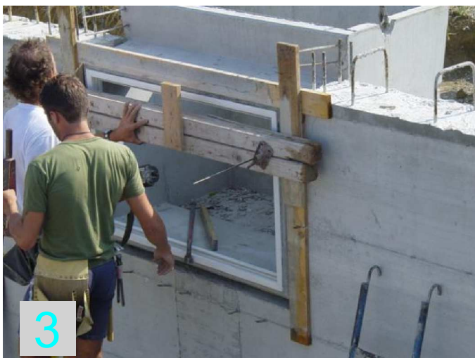
3 Fissaggio della Bocca di Lupo alla parete utilizzando i 4 tondini predisposti e morsetti.
