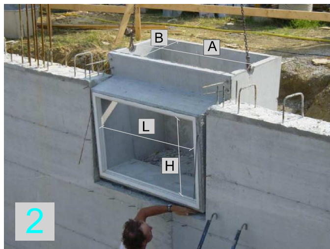
2 Sollevamento e posizionamento della Bocca di Lupo con catene agganciate ai ferri predisposti.
